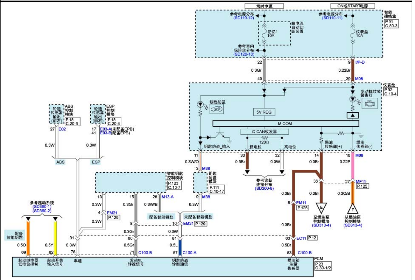
发动机控制系统(G4KH : THETA-II 2.0L T-GDI)(8)
